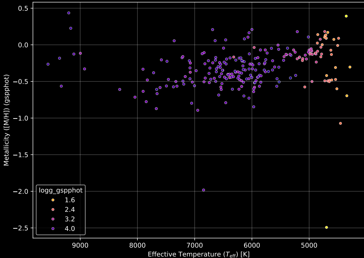
GALAH DR4 Field: [8489] Stellar Population Parameters (n= 234)
