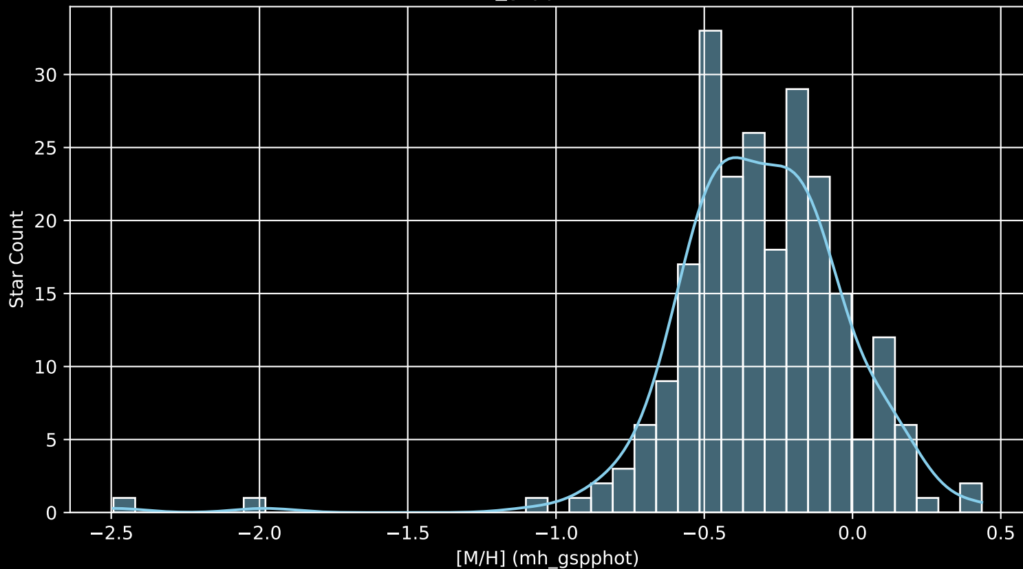
GALAH DR4 Field: [8489] [M/H] (mh_gspphot) (n= 234)
