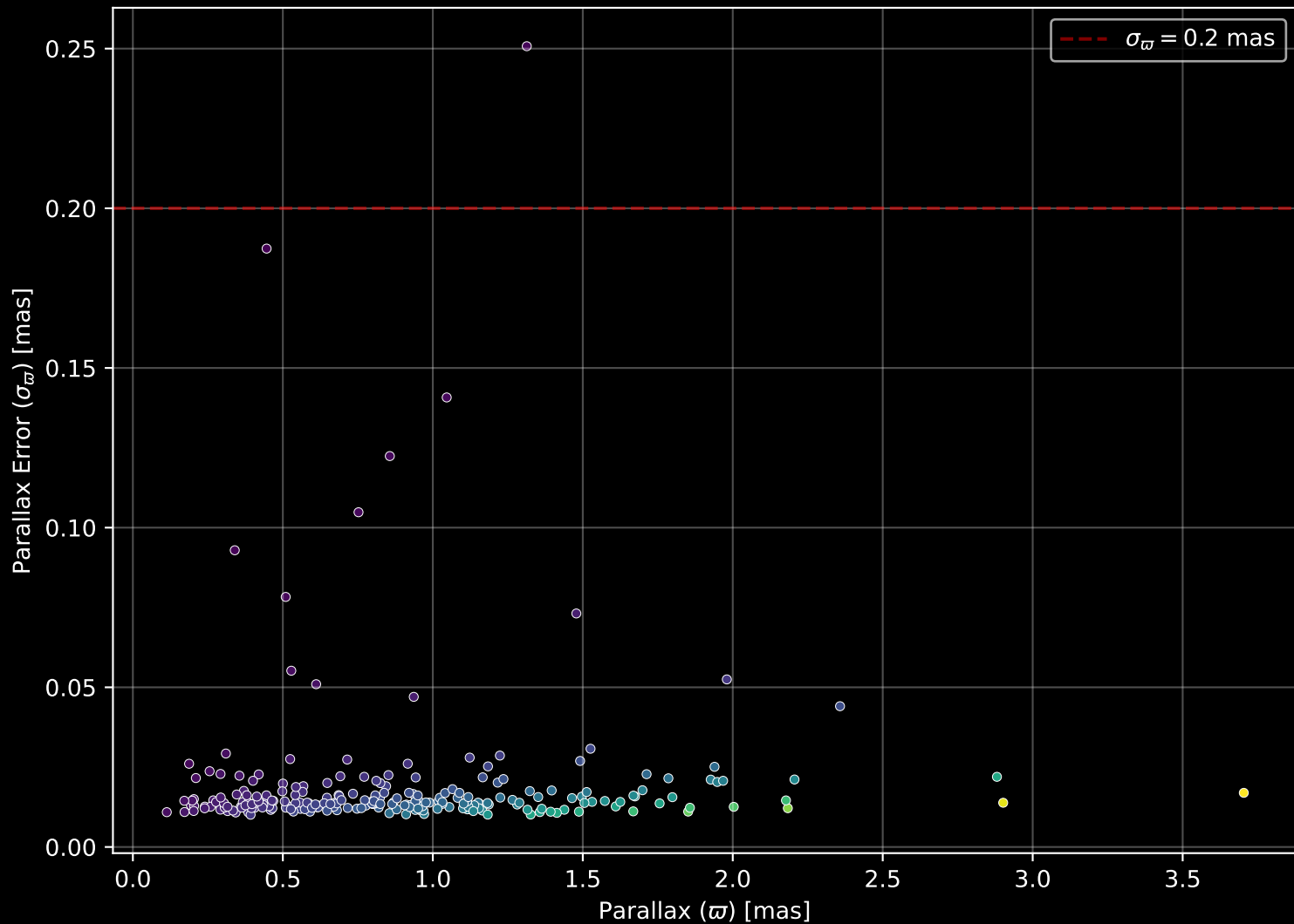
GALAH DR4 Field: [8489] Parallax Quality (n= 234)
