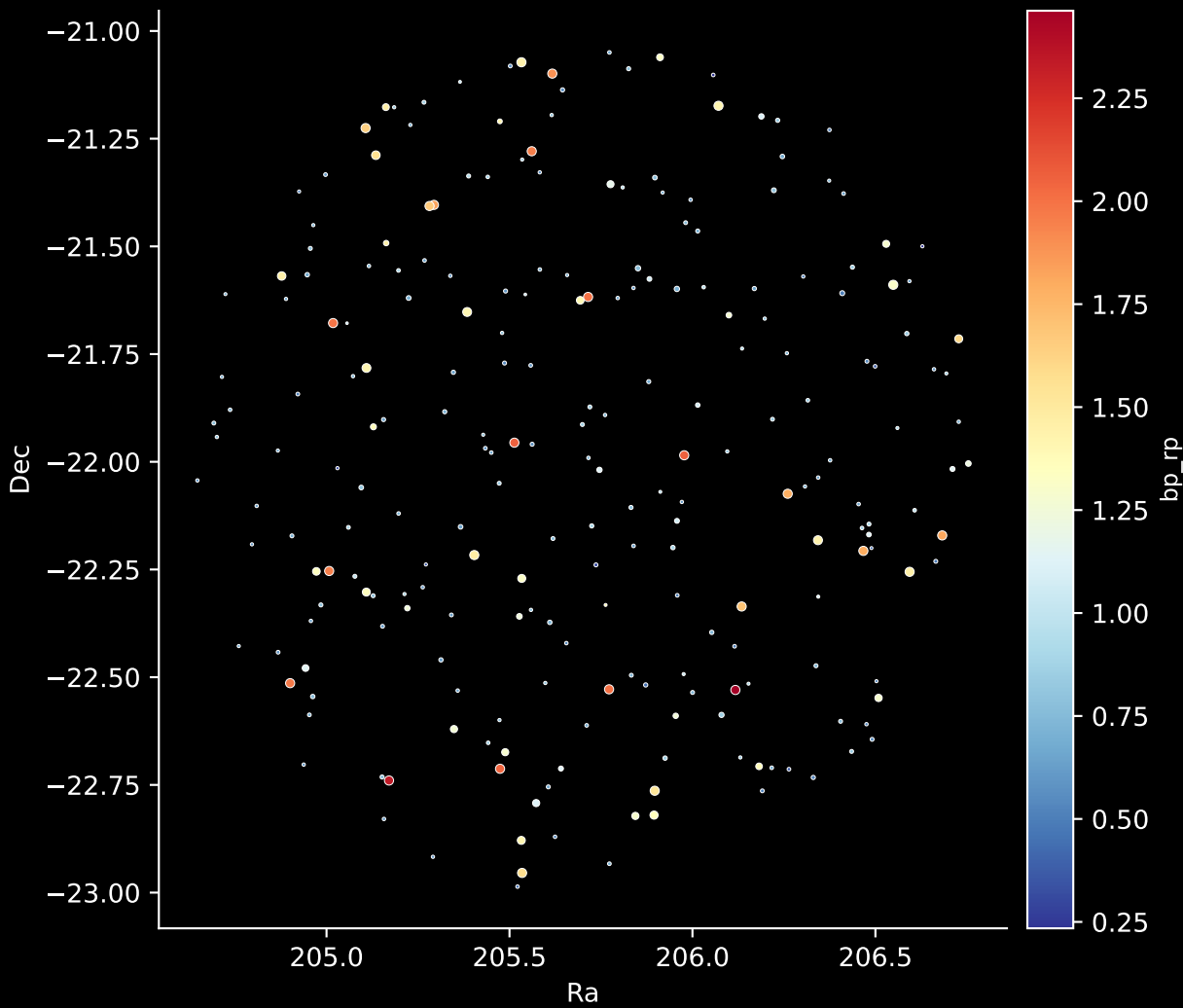
GALAH DR4 Field: [8489] Stars: 234
